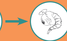
pupa
